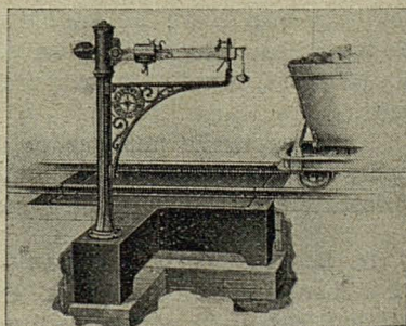
Báscula model 250' per a pesar vagonets
