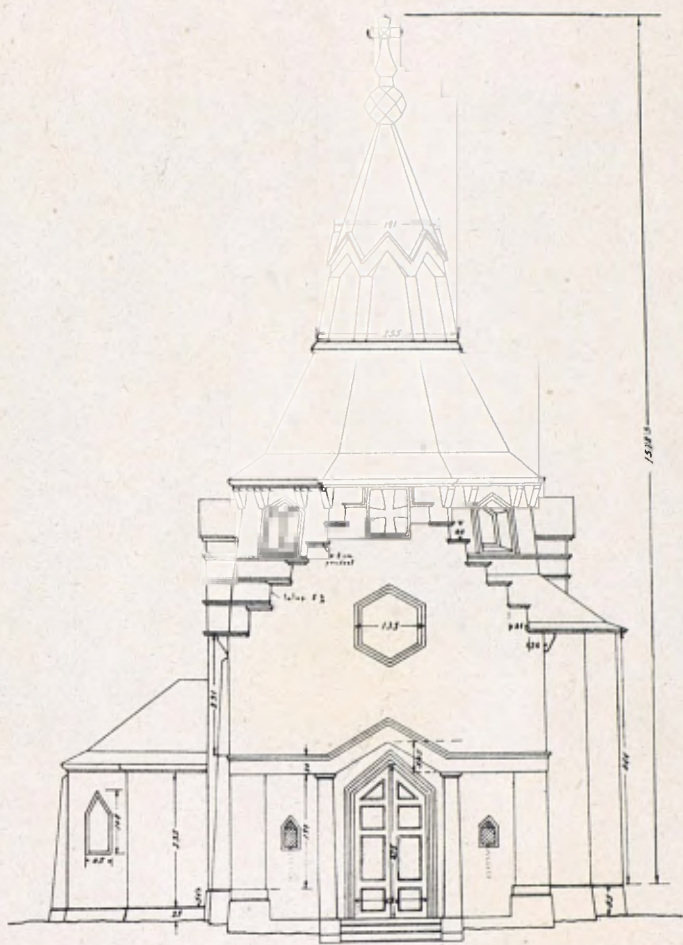
Projecte d'Ermida dedicada a Sant Antoni en el tossal de Serc (Lleida). En construcció. Joan Bergós, arquitecte.
