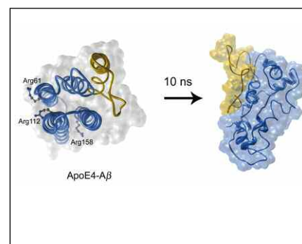
Desestabilització estructural del complex format per ApoE4 (blau) i el pèptid beta amiloide (daurat).
