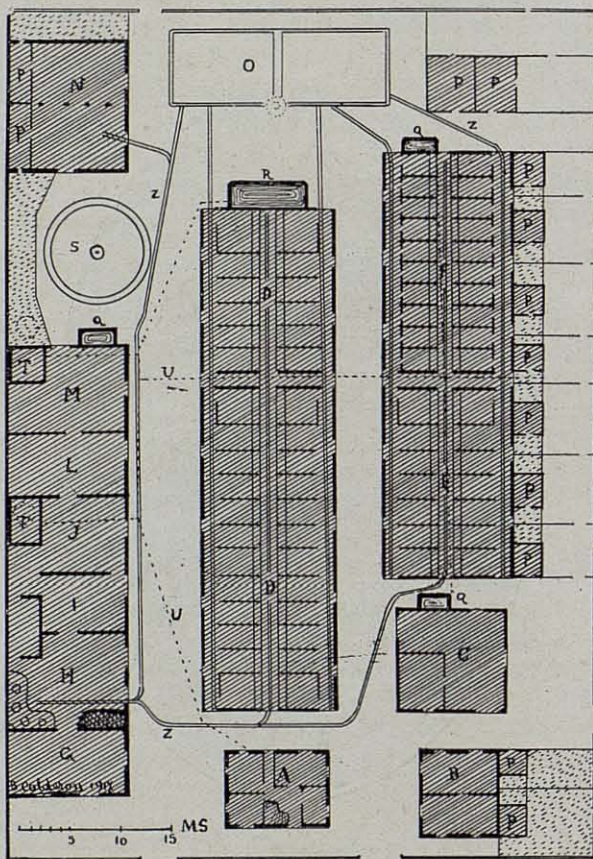
Plano de la disposición de los edificios de una hacienda de cierta importancia: A, casa habitación; B, despacho, almacén de semillas, frutero, etc.; C, cochera, almacén para maquinaria, taller y otros servicios; D, establos; E y F, cuadras y cochideras, G y H, comedor y alojamiento del personal; I y J, depósito de carbón, lavadero, molino, corta-raíces y otros servicios; L y M, almacenes de tubérculos y raíces; N, almacén de heno; O, estercolero; P, gallineros con sus parques; Q, pilas; R, baño; S, malacate; T, depósitos elevados de agua; U, conductos de agua; Z, vía férrea; MS, escala de metros.
