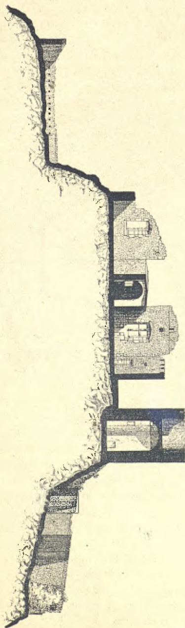
CASTELL DE BURRIACH. — SECCIÓ A B (ESCALA DE 1 PER 400)
