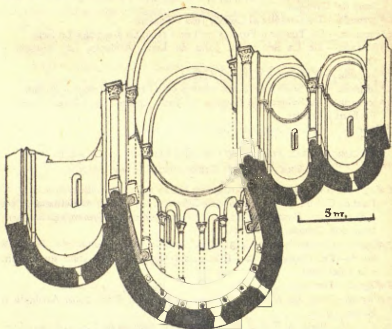
Planta de l'absis de Sant Pere de Galligans
