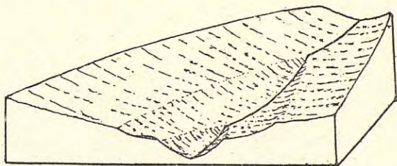
Esquema explicatiu de l'encaixament dels cicles d'erosió, segons Baulig
