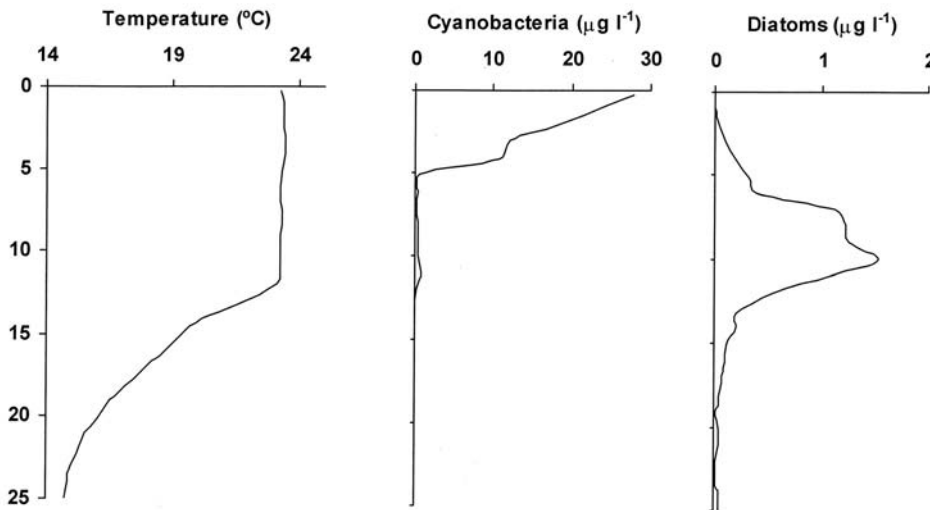
Figure 5. Vertical distribution of temperature (°C), Cyanobacteria biomass ( \mu\text{g l}^{-1} ) and Diatoms biomass ( \mu\text{g l}^{-1} ) during the late summer 2003 extensive survey in El Gergal reservoir. Distribución vertical de temperatura (°C), biomasa de Cianobacterias ( \mu\text{g l}^{-1} ) y biomasa de Diatomeas ( \mu\text{g l}^{-1} ) en el embalse de El Gergal durante el muestreo extensivo llevado a cabo a finales de verano de 2003.
