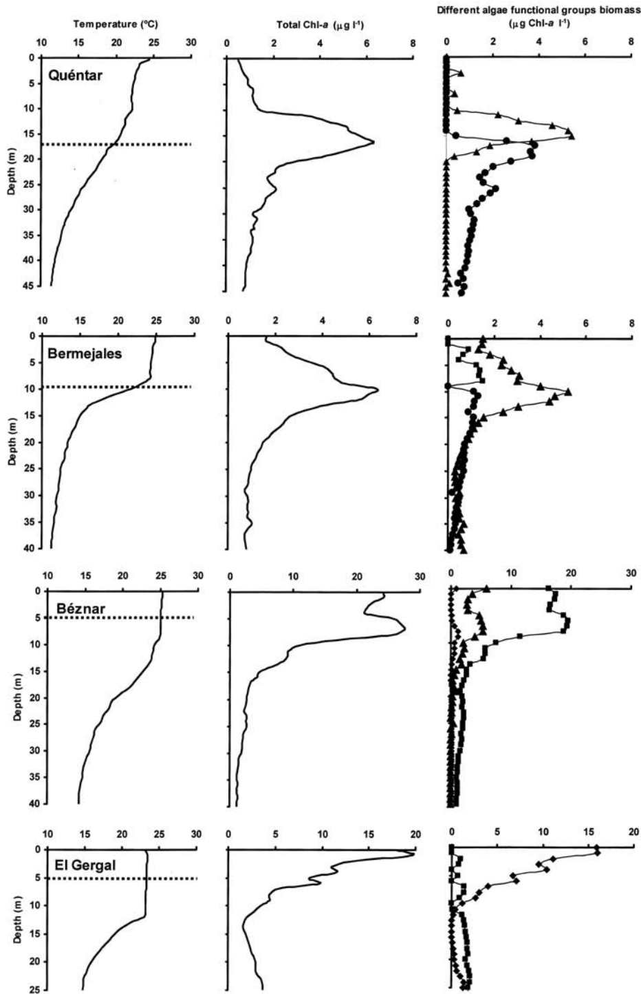
Figure 3. Vertical distribution of temperature (left), total Chl-a (centre) and different phytoplankton functional groups (right) in the studied reservoirs. Horizontal dotted line represent the euphotic layer depth. Distribución vertical de la temperatura (izquierda), Chl-a total (centro) y distintos grupos funcionales del fitoplancton (derecha) en los embalses estudiados. La línea de puntos horizontal representa la profundidad de la zona eufótica.
