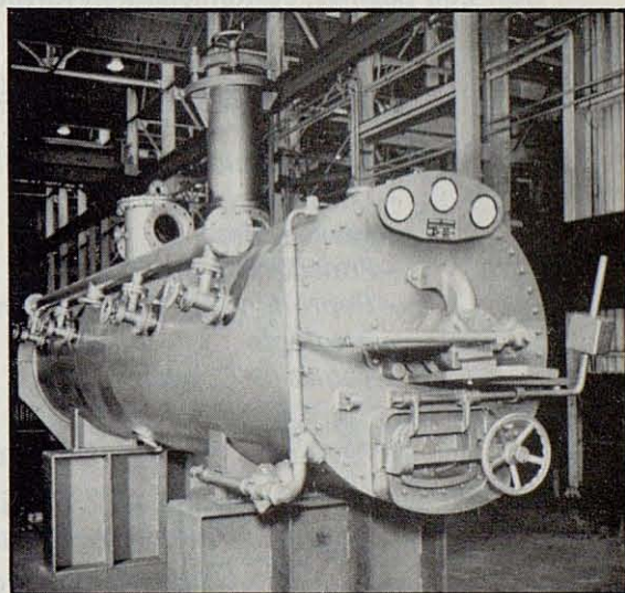
DIGESTOR «SD-50»
