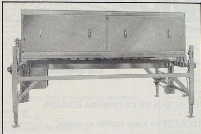
DESPLUMADORA «DURA 2»
