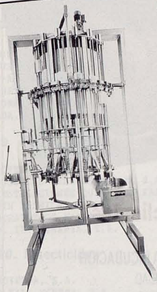
Extractor de buches para pavos
