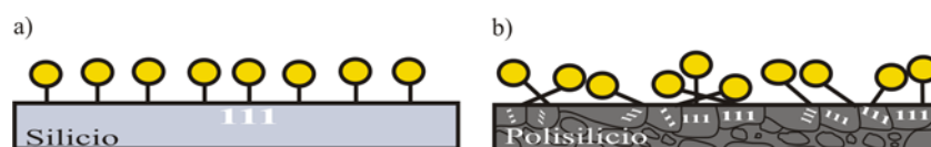
Figura 5. Crecimiento de los nanohilos en la dirección \langle 111 \rangle , a) sobre silicio monocristalino de forma alineada y b) sobre polisilicio de forma desalineada.
