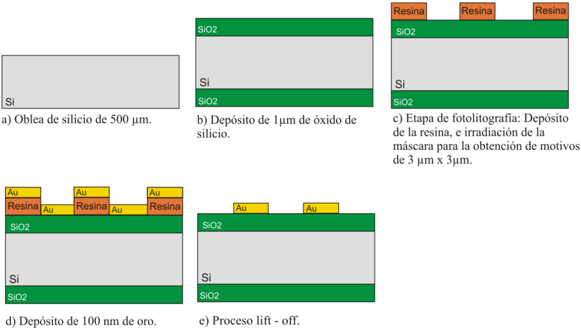
Figura 12. Secuencia de pasos para la fabricación de microchips de oro.
