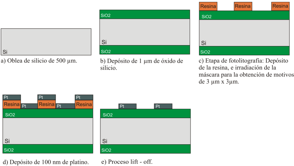
Figura 15. Secuencia de pasos para la fabricación de microchips de platino.
