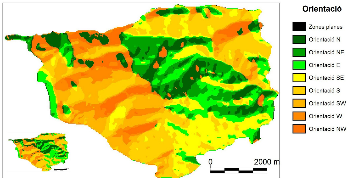
Figura A.4: Mapa d'orientacions (imatge gran amb 9 orientacions, imatge petita amb 5 orientacions). Elaboració pròpia a partir del MDE
