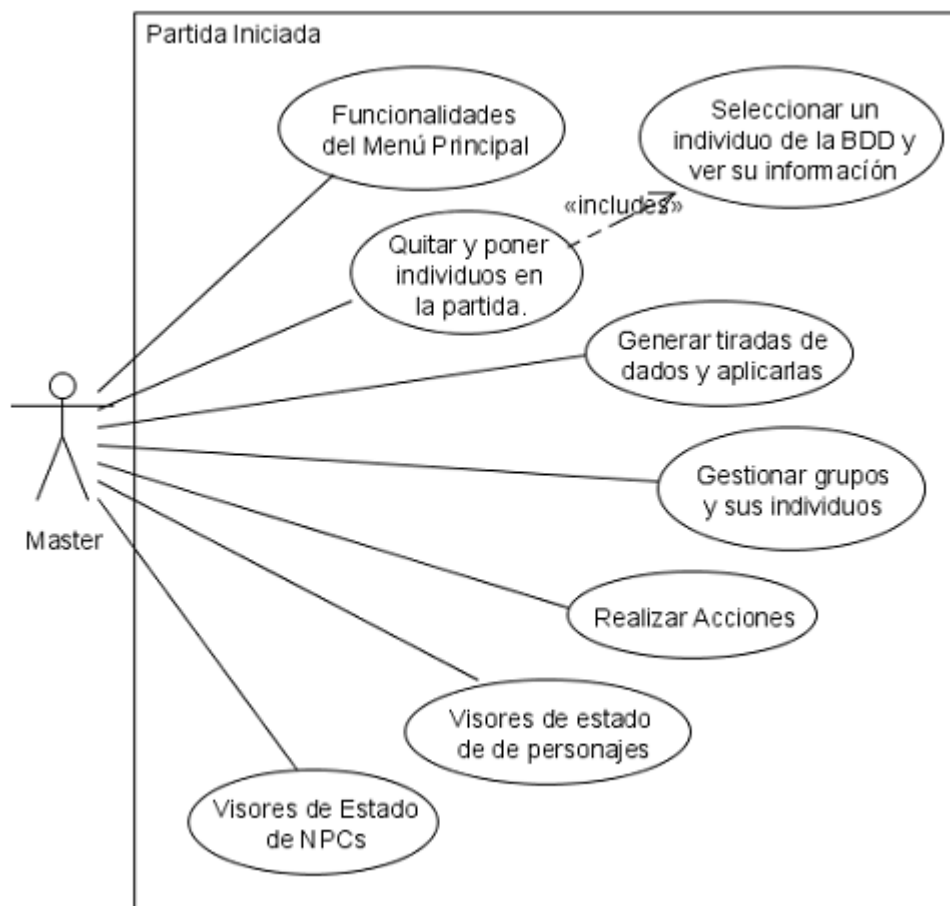
Figura 4.2: Casos de uso partida
