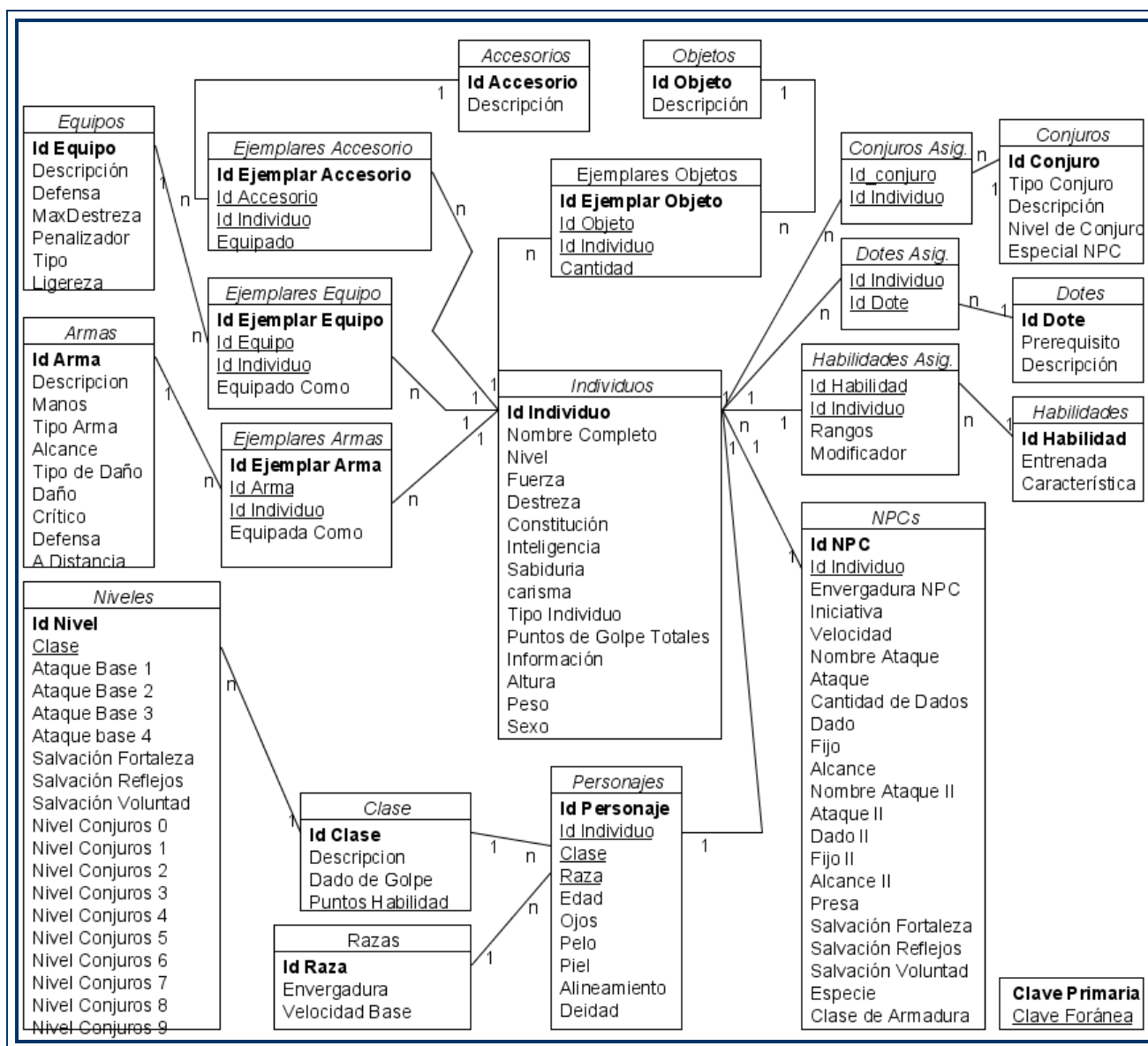
Figura 3.3: Base de Datos
