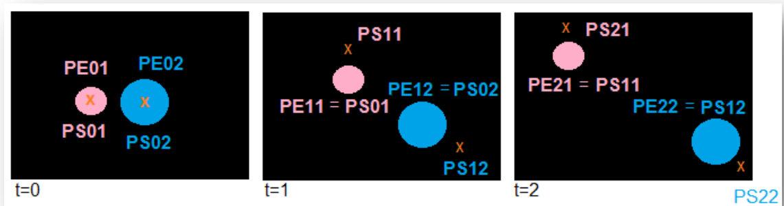
Figura 21: Correspondència entre paràmetres d'entrada i de sortida de Filtre de Kalman.
