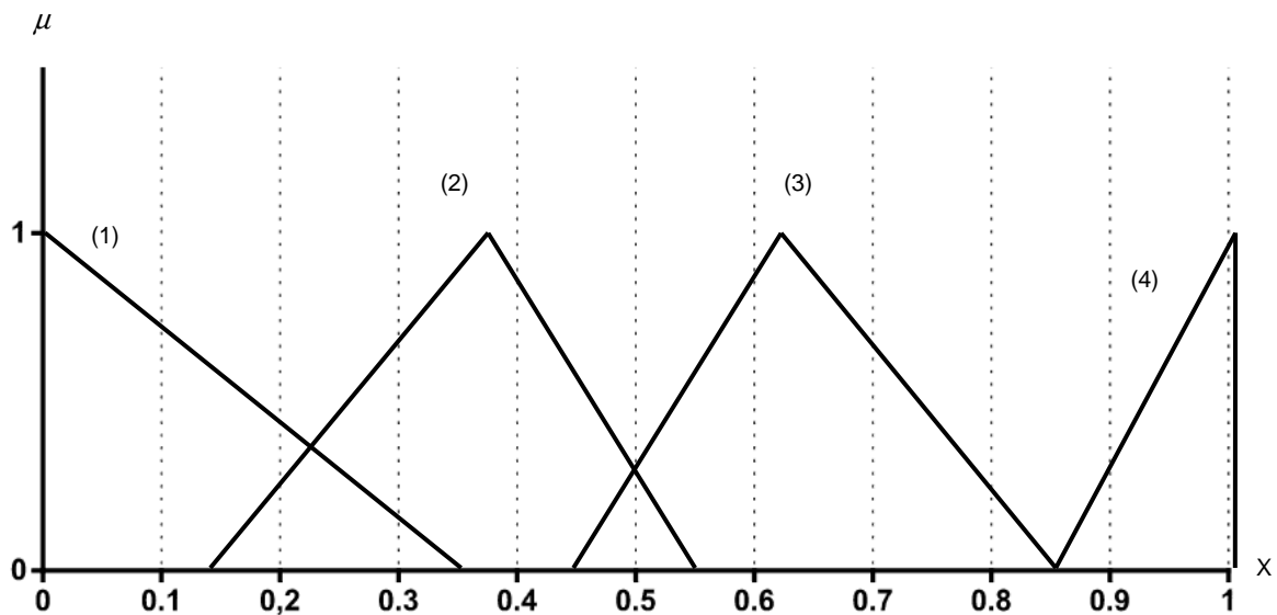
Figura 3.8: Conjunt de funcions de pertinença de fricció.
