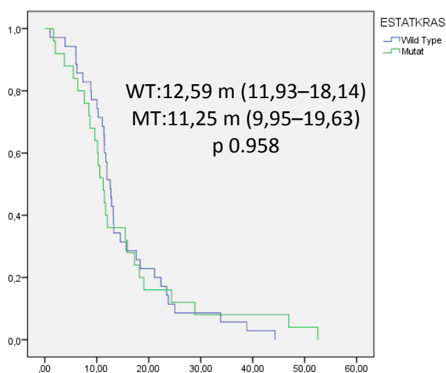
Gràfic 2: SLP en funció d'estat de KRAS
