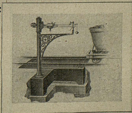
Bàscula model 253 per a pesar vagonetes
