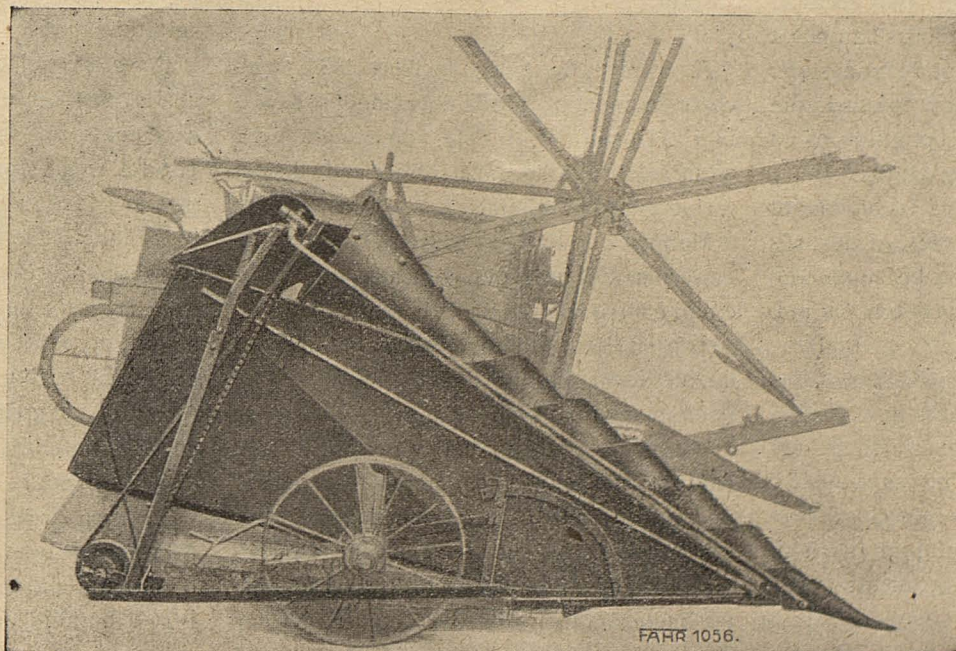
Figura 2.—Detall de la part principal de l'aparell que aixeca els sembrats ajeguts. Es tracta d'una espiral sense fi, rotativa que de la mateixa manera que rodant aixeca el sembrat de l'exterior, el situat a l'interior el posa en condicions de caure bé a la plataforma per tal que vagi ben aparellat
