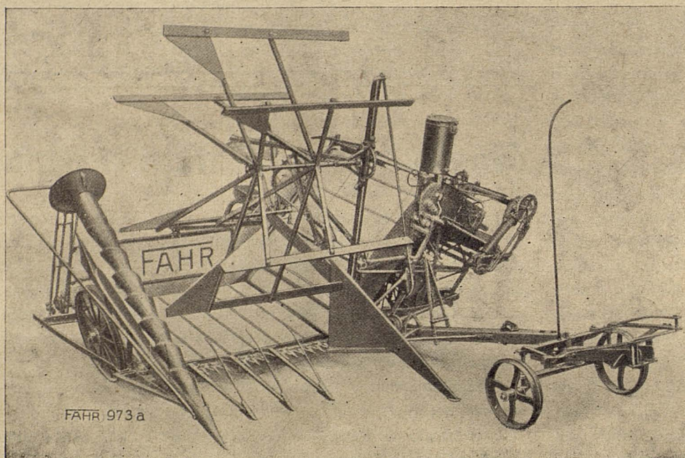
Figura 1.— Segadora lligadora, amb l'aditament especial per a segar el blat bolcat, que és un torn sense fi, situat a l'esquerra del gravat. A primer terme s'hi veu un avant-tren, conduït per dues rodes, que no té cap relació amb l'aparell objecte d'aquest article, però que resulta de gran utilitat i és molt recomanable la seva adaptació a tota classe de segadores i lligadores, doncs té per finalitat que el pes de la màquina no graviti damunt els animals de tracció, facilitant a l'ensems, de poder girar més fàcilment
