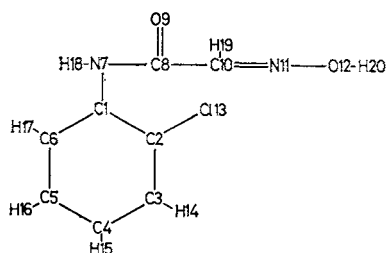
Fig. 1. — Fórmula desarrollada de la 2-cloro isonitrosoacetanilida.
