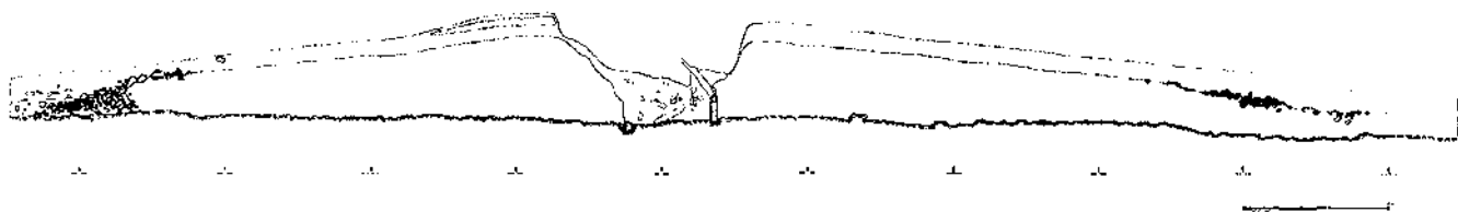
Fig. 2. Secció longitudinal de l'estructura tumular de Font de la Vena. Entre el nivell superficial i l'únic que conforma el túmul s'aprecia la bossada de les terres provinents de l'interior de la cambra, resultat de la seva violació. És d'aquest nivell que es recuperà la gran majoria de material lític. El sector W presenta únicament la part superficial de l'anell/cromlec.
