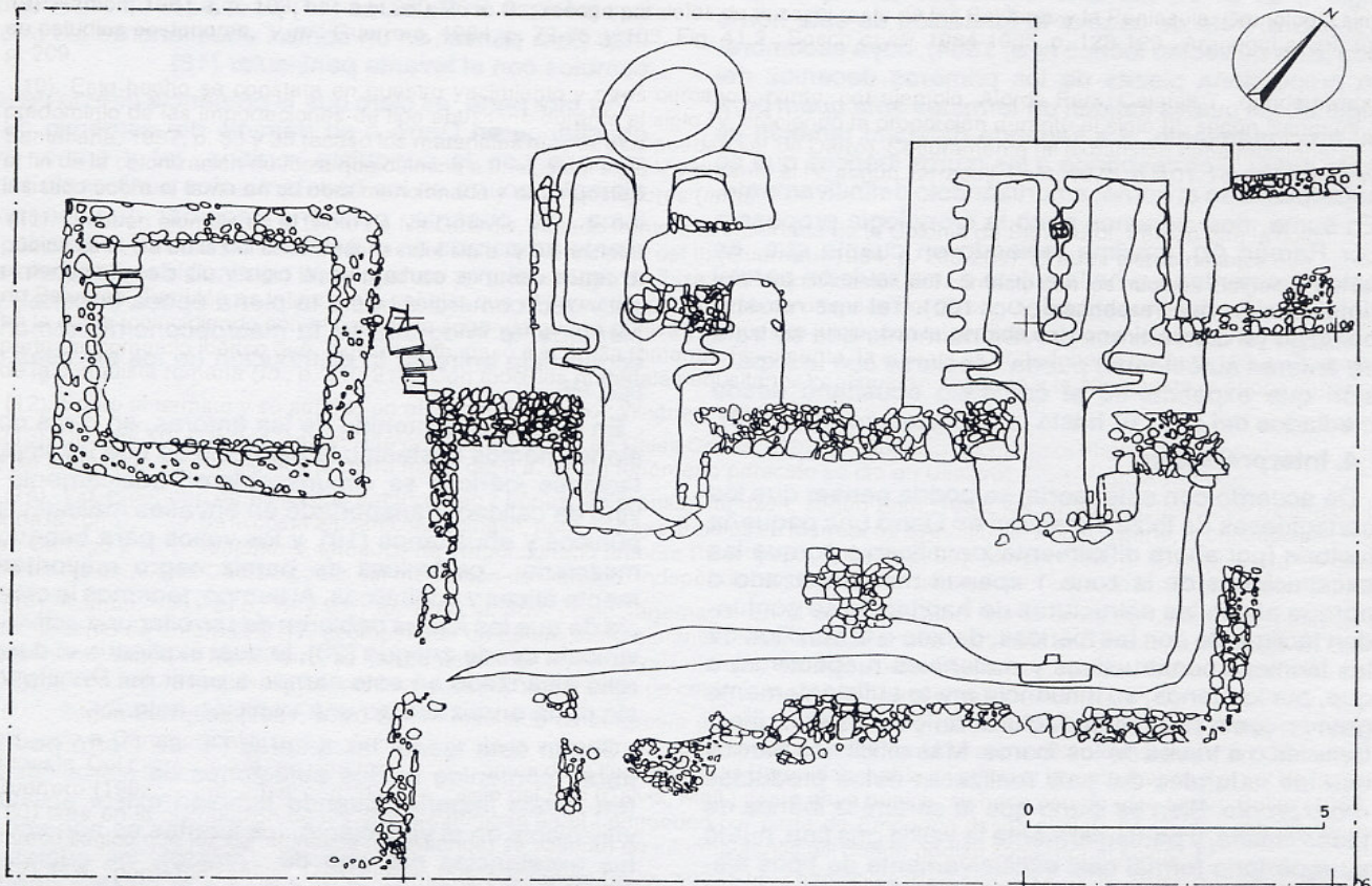
Figure 4 - Planta del taller de ánforas del siglo I.
