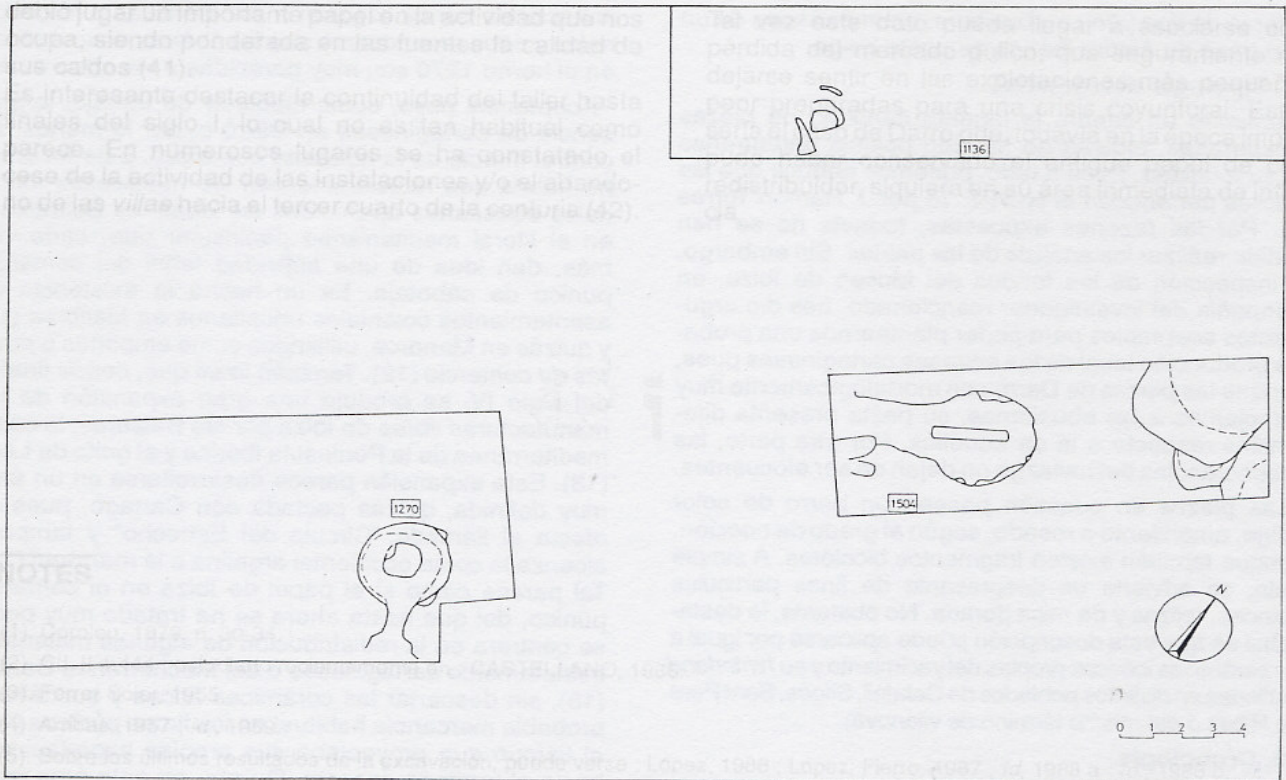
Figure 3 - Planta de los hornos que produjeron las cerámicas ibéricas (u.e. 1136, 1504) y las ánforas de tipo PE (u.e. 1270).
