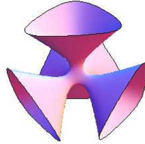
Superficie de Clebsch: x^3 + y^3 + z^3 + 1 - (x + y + z + 1)^3 = 0 , d = 3, \quad (3m^2 - 3m + 6)/2 .
