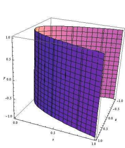
Cilindro parabólico: z^2 - x = 0
