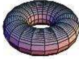
Figura 1.2: El 2-toro y una expresión algebraica del mismo.
