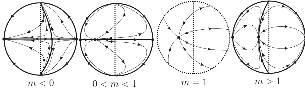
Figura 6.8: Retratos de fase del sistema (6.27). Ellos tienen infinitas separatrices.
