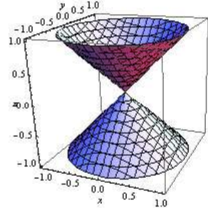
Cono: x^2 + y^2 - z^2 = 0
