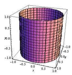
Cilindro elíptico: x^2 + z^2 - 1 = 0
