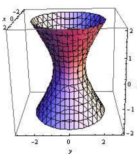
Hiperboloide de una hoja: x^2 + y^2 - z^2 - 1 = 0
