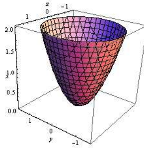
Paraboloide elíptico: y^2 + z^2 - x = 0
