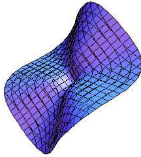
Cúbica de Fermat: x^3 + y^3 + z^3 = 1 , d = 3, \quad (3m^2 - 3m + 2)/2 .
