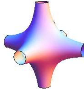
Superficie Racor: x^2y^2 + x^2z^2 + y^2z^2 = 1 , d = 4, \quad 2m^2 - 4m + 6 .
