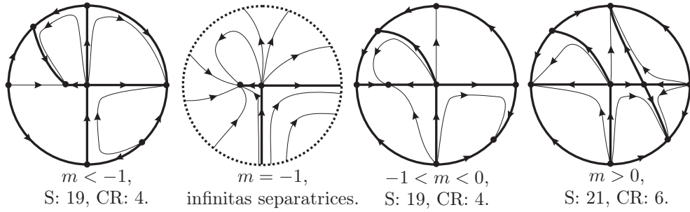
Figura 6.16: Retratos de fase del sistema (6.45).
