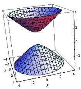
Hiperboloide de dos hojas: x^2 + y^2 - z^2 + 1 = 0
