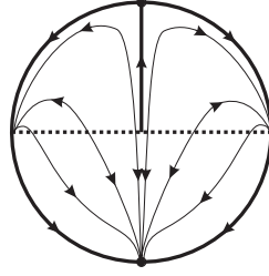
Figura 6.2: Retrato de fase del sistema (6.11) cuando b \neq 0 . Posee infinitas separatrices.
