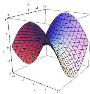
Paraboloide hiperbólico: y^2 - z^2 - x = 0
