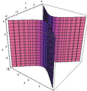
Cilindro hiperbólico: x^2 - z^2 - 1 = 0
