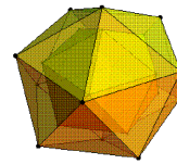
(d) Two icosahedra
