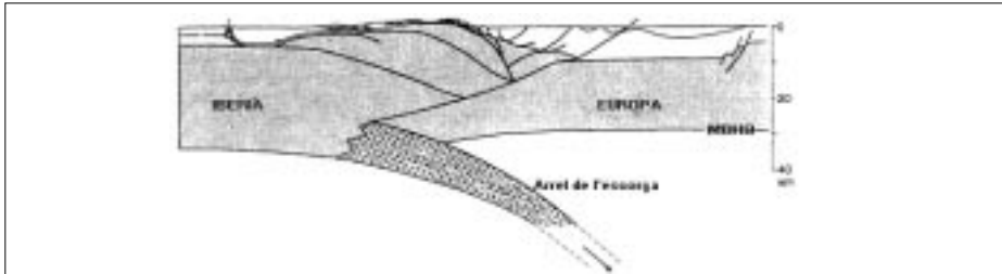
Esquema d'una secció transversal de l'escorça sota els Pirineus a la zona centre-oest de la serralada.
