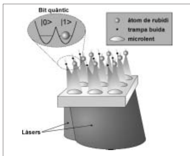
Esquema simplificat del dispositiu experimental en què es basa el computador quàntic.
