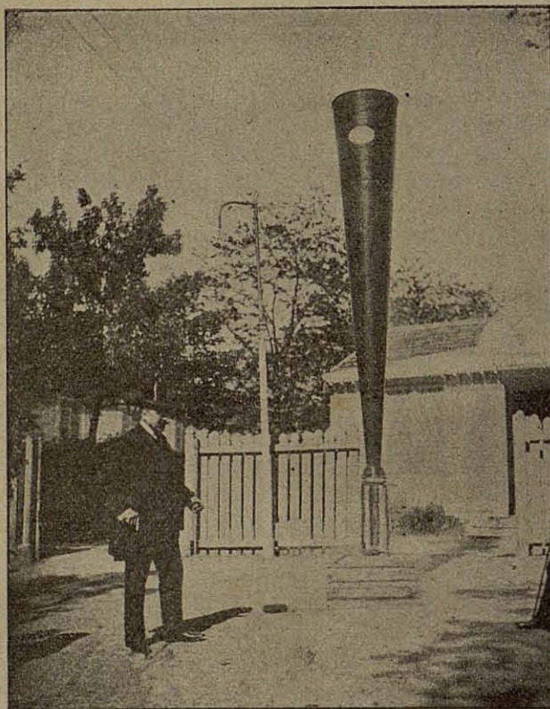
El Ministro de Agricultura D. José Canalejas disparando un cañón granicifugo sistema Bori, emplazado en los Jardines de la Exposición
