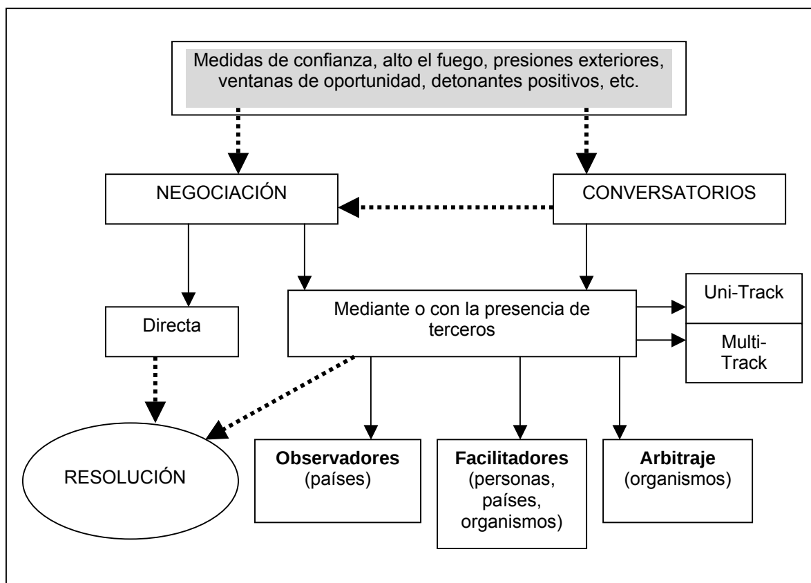
Gráfico 3.1. Esquema habitual de un proceso de negociación
