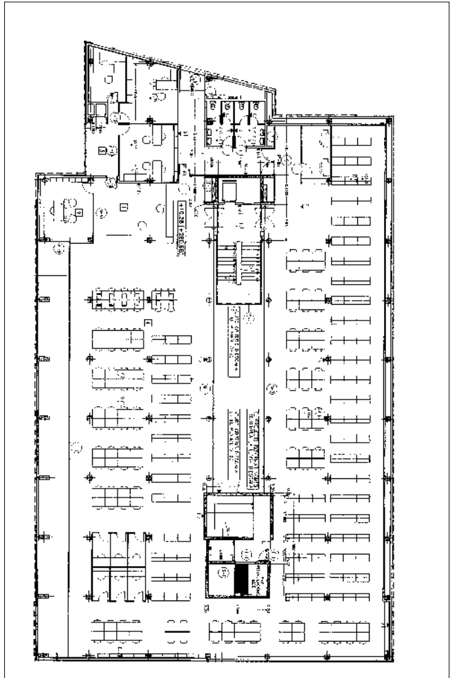
Biblioteca i Hemeroteca General. Planta nivell 3.
