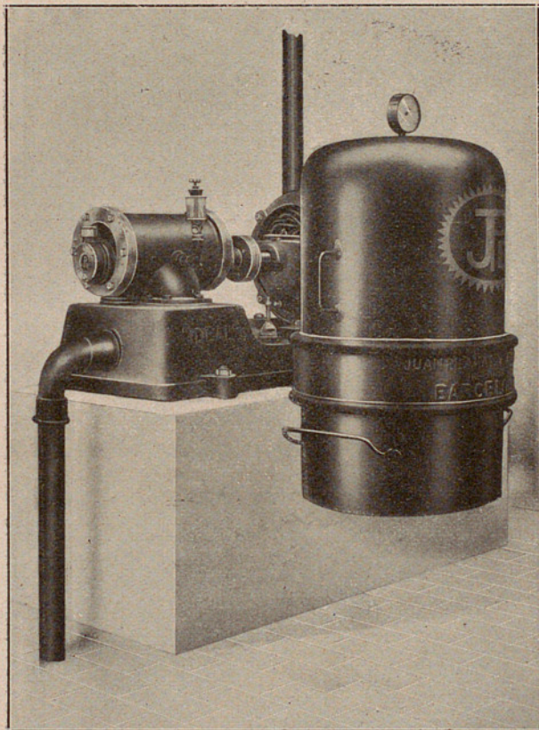
GRUPO ELECTRO-ASPIRADOR CON FILTRO PARA EL POLVO
