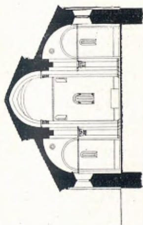
SECCIÓ TRANSVERSAL
