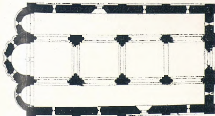
PLANTA RESTAURADA
