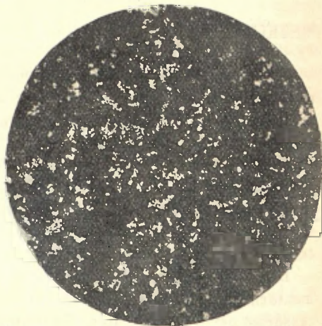
Fig. 4—Repartició de ferre niquelífer per reflexió en el meteorit de Girona ( \times 4 )
