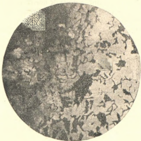
Fig. 3.—Microfotografia del meteorit de Canyelles ( \times 30 )
