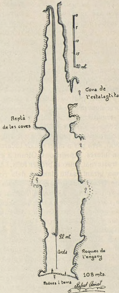
Avenç de la Sibinota.—Tall longitudinal
