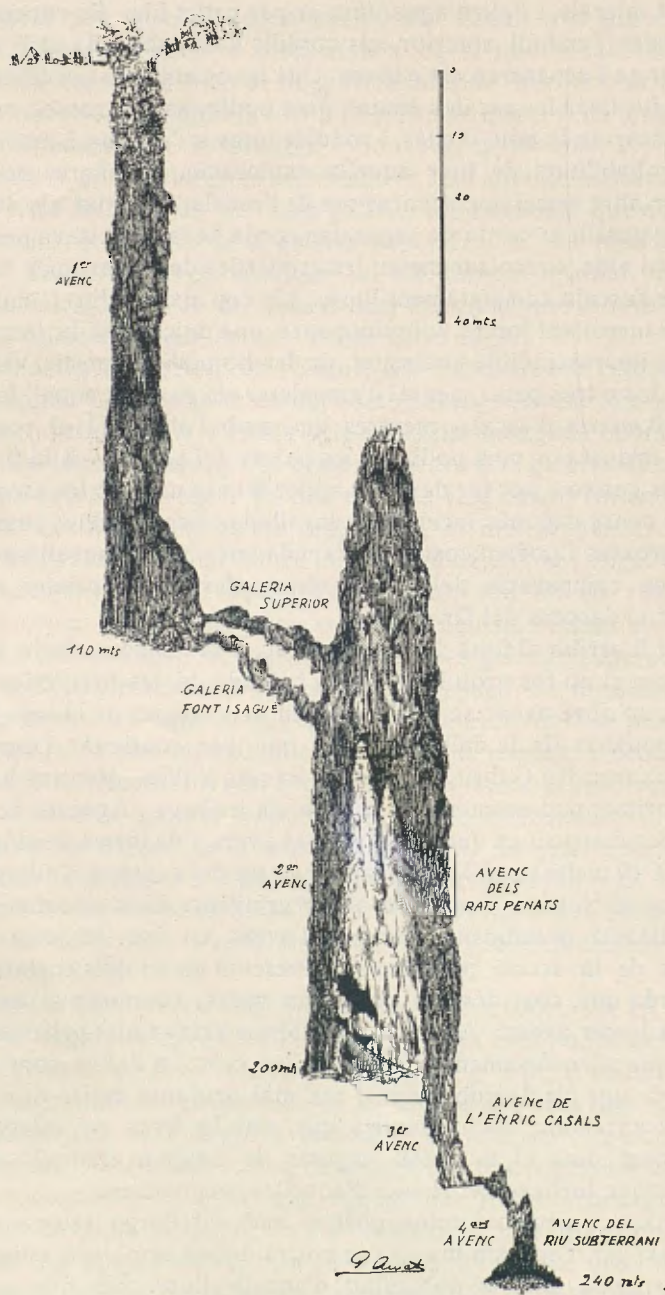
Avenç de la Ferla. — Secció longitudinal.
