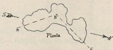
Avenc de les Terradelles. Secció longitudinal i planta.
