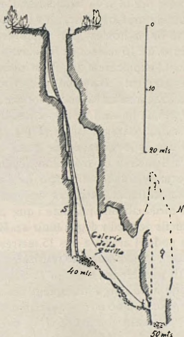
Avenc del Corral Nou.
