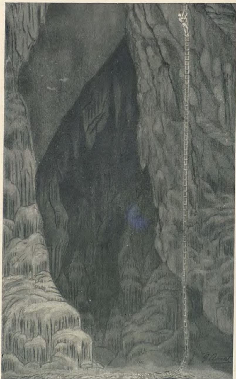
AVENC DE CAN SADURNÍ. - VISTA DE CONJUNT.
