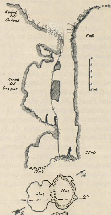
Avenc de la Fragata.
