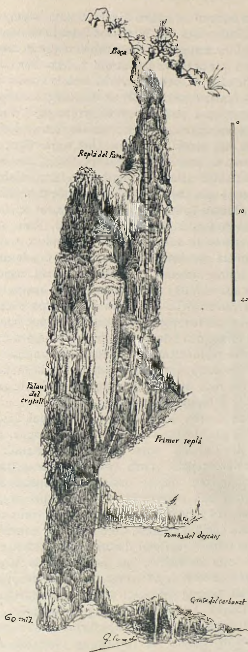
Avenc de l'Arcada. - Secció longitudinal.
