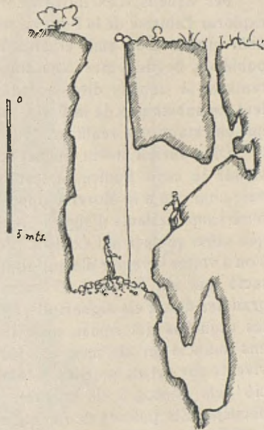
Avenc del Campgràs.
