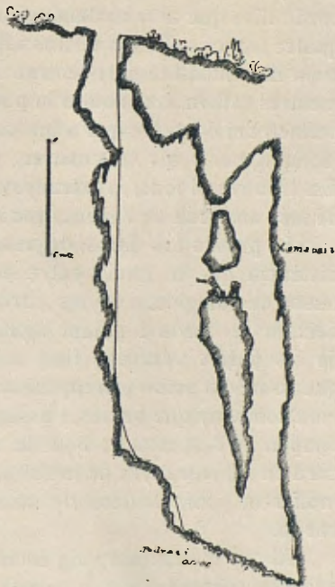
Avenc del Clos.
