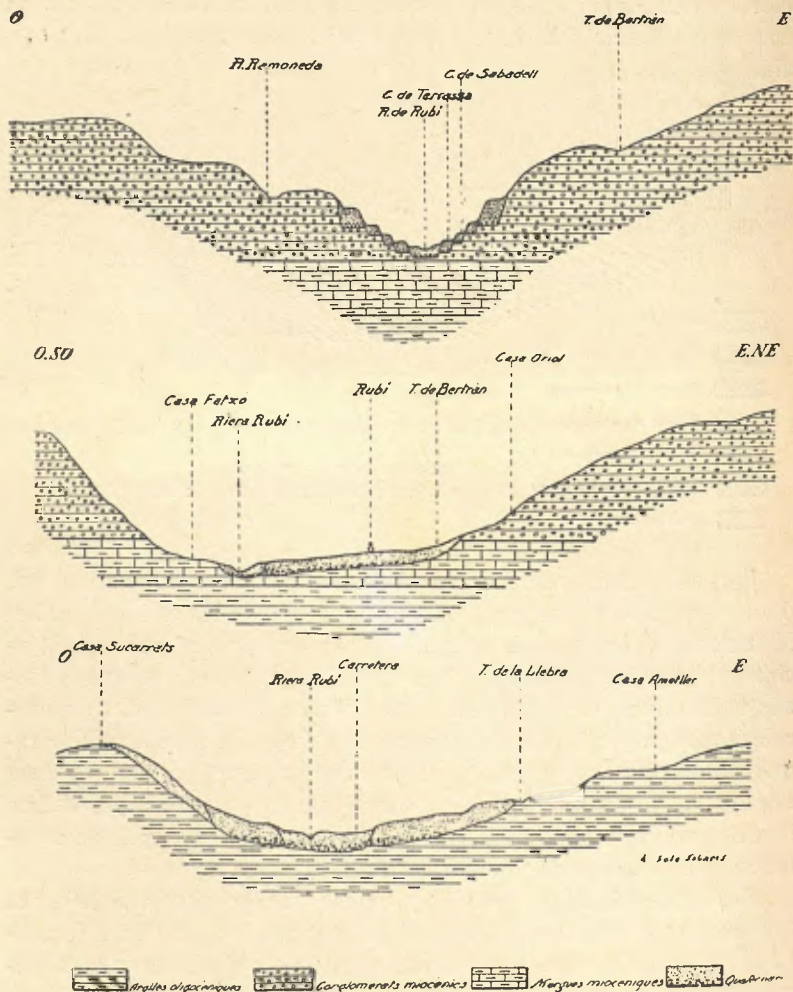
Talls seriat a la riera de Rubí, per mostrar l'excavació de la seva vall en les diferents capes del Vallès
