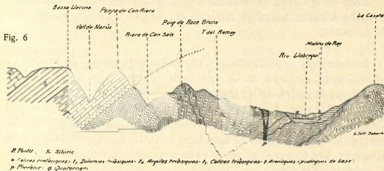
Tall de la vall del Llobregat, a Molins de Rei
