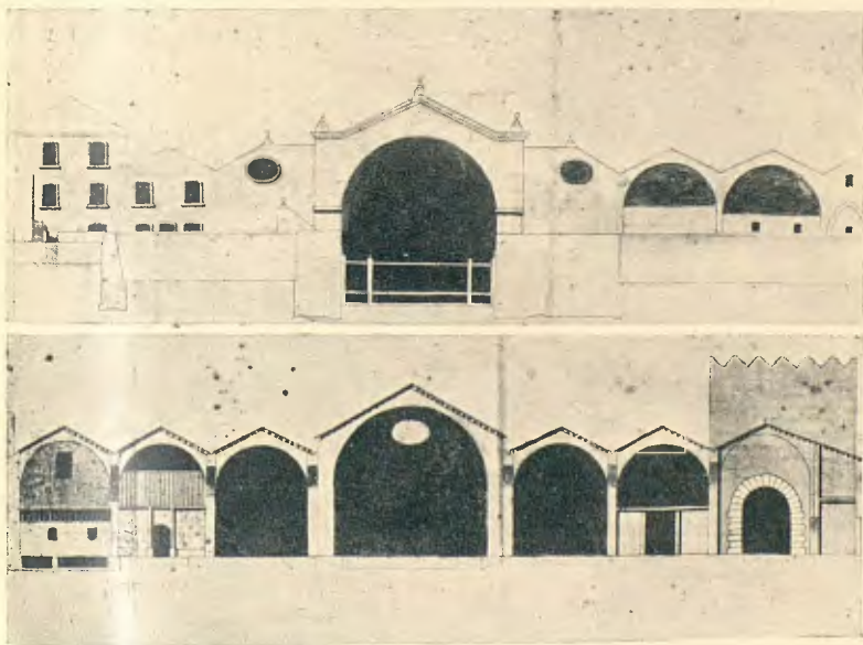
SEGLE XVII : PERFIL DE LES DREÇANES EXISTENT A L'ARXIU MUNICIPAL
