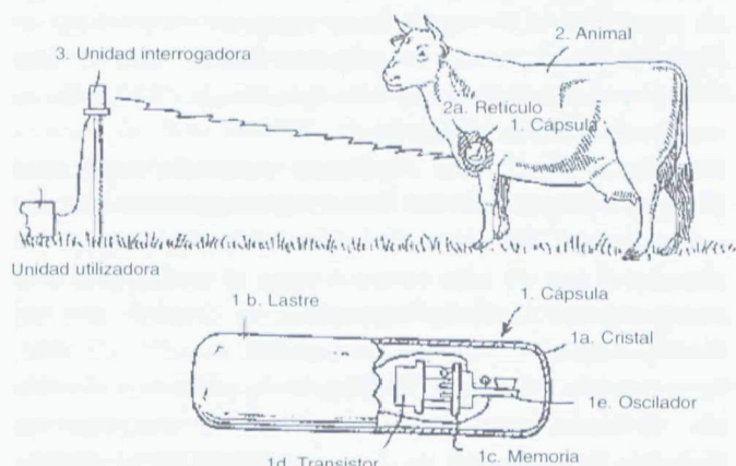
Figura 1. Primer sistema de identificación electrónica en ganado bovino (Hanton y Leach, 1974).
