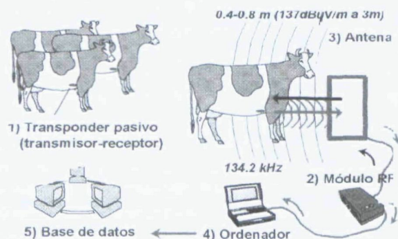
Figura 2. Esquema de un sistema completo de identificación electrónica en ganado bovino (Caja, 1996).
