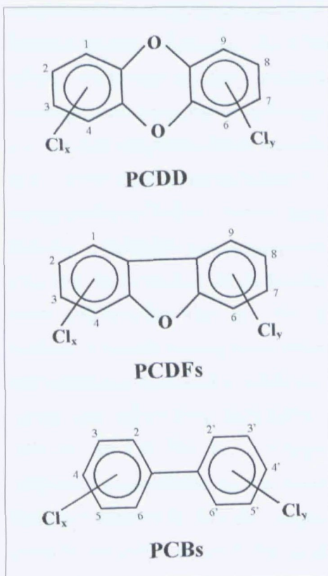
FIGURA 1. Estructura bàsica i numeració dels anells en PCDDs, PCDFs i PCBs.
