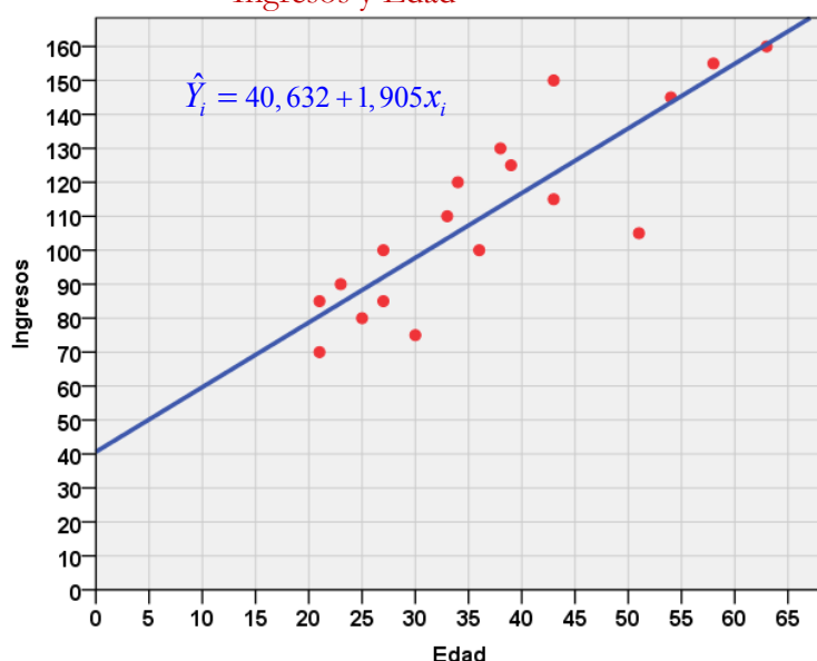
Gráfico III.9.14. Gráfico de dispersión de la regresión entre Ingresos y Edad
