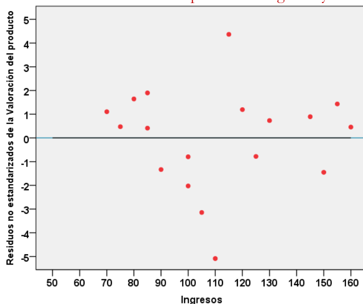
Gráfico III.9.20. Diagrama de dispersión entre los residuos no estandarizados de la Valoración y las variables independientes Ingresos y Edad
