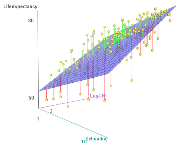
Gráfico III.9.19. Gráfico de dispersión de la Esperanza de vida según los años de escolarización y la renta per cápita transformada
