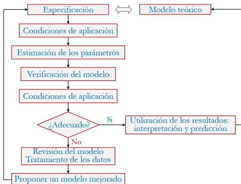
Gráfico III.9.9. Esquema del proceso de un análisis de regresión
