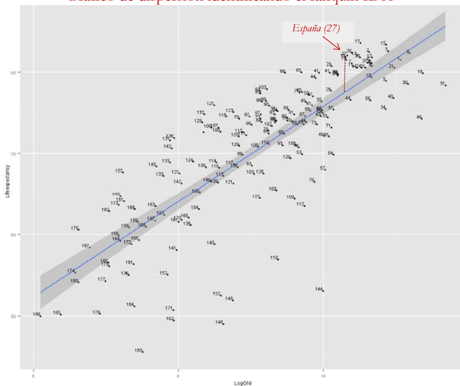
Gráfico de dispersión identificando el ranquin IDH 18
