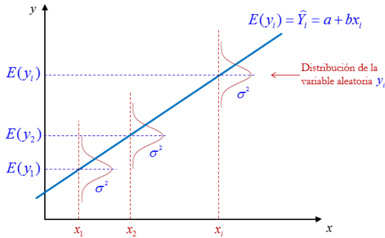
Gráfico III.9.12. Condiciones de aplicación de la regresión. Distribución de los errores
