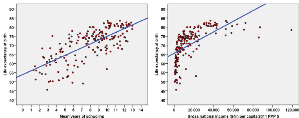
Gráfico III.9.15. Gráficos de dispersión de la regresión entre la Esperanza de vida al nacer y los Años de escolarización y la Renta per cápita
