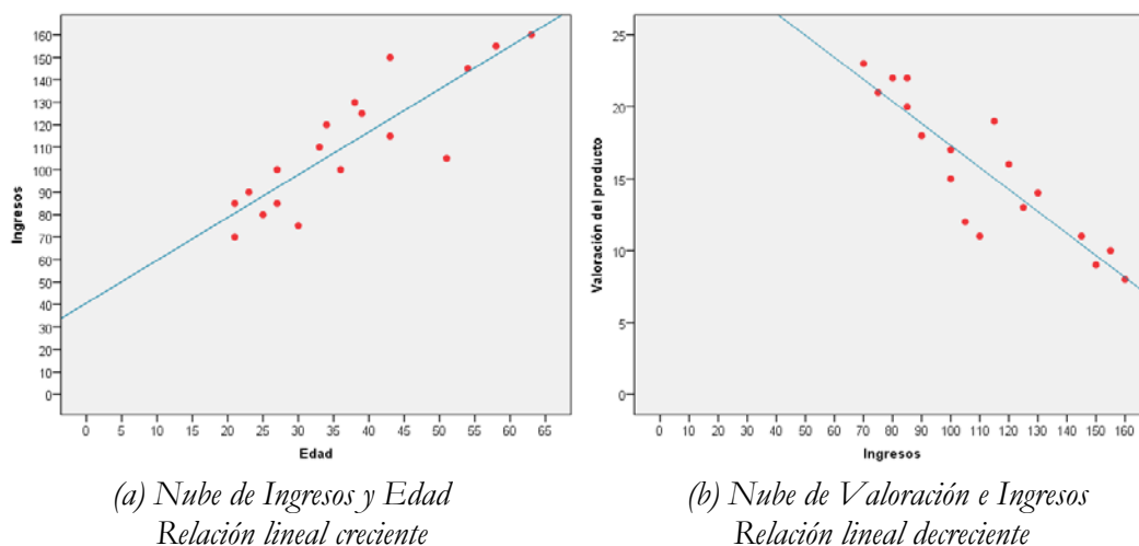
Gráfico III.9.3. Diagramas de dispersión con las nubes de puntos
