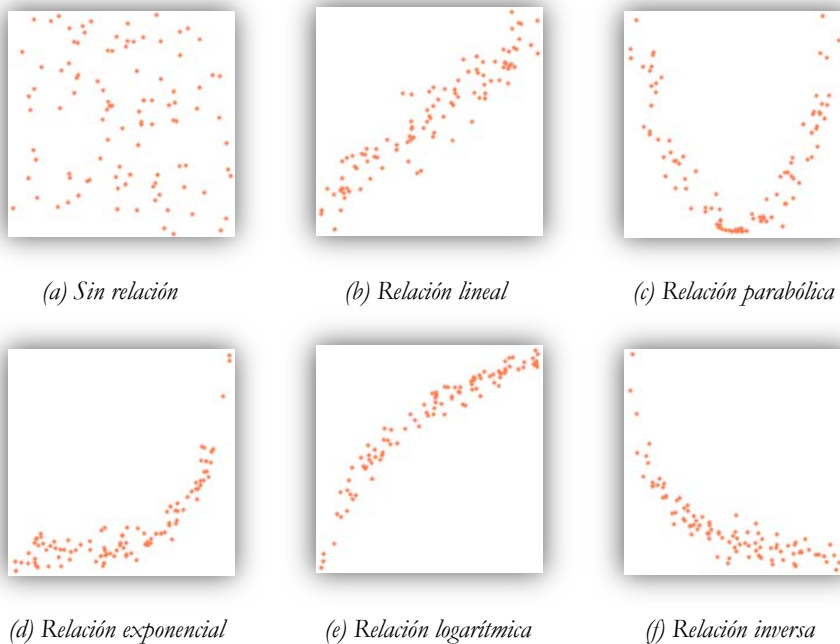
Gráfico III.9.6. Diagramas de dispersión y funciones de relación
