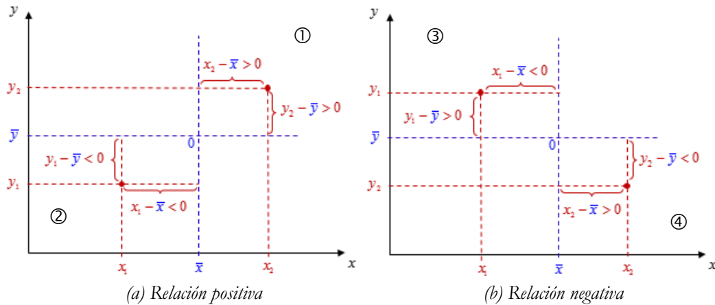
Gráfico III.9.4. Representación de la covariación
