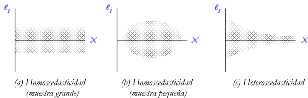
Gráfico III.9.22. Representación gráfica de la varianza de los errores
