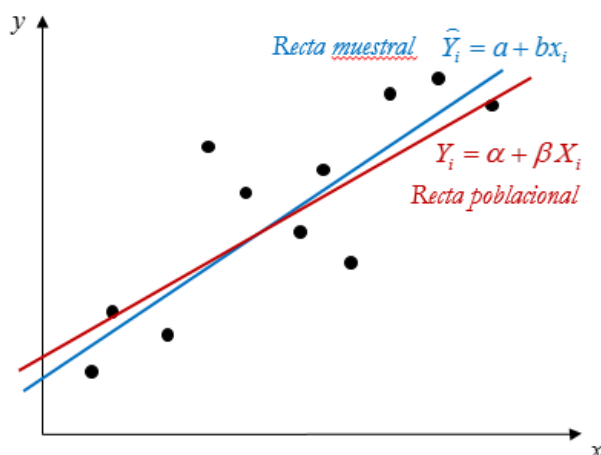
Gráfico III.9.11. Recta de regresión muestral y poblacional
