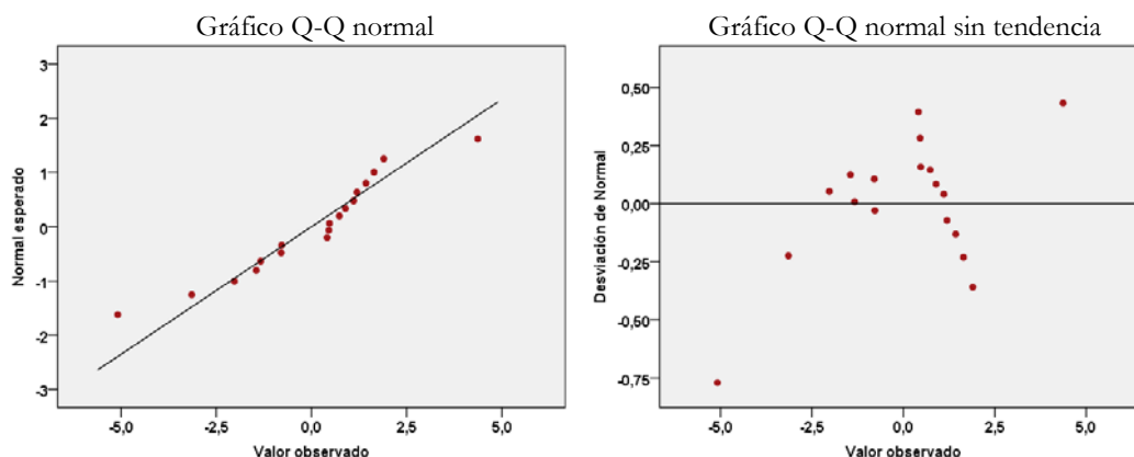
Gráfico III.9.21. Gráficos de probabilidad normal Q-Q de los residuos. Valoración del producto según Edad e Ingresos
