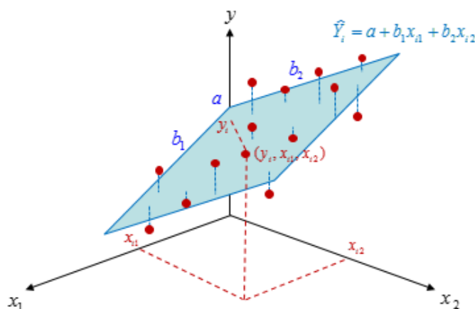
Gráfico III.9.18. Modelo lineal de regresión múltiple
