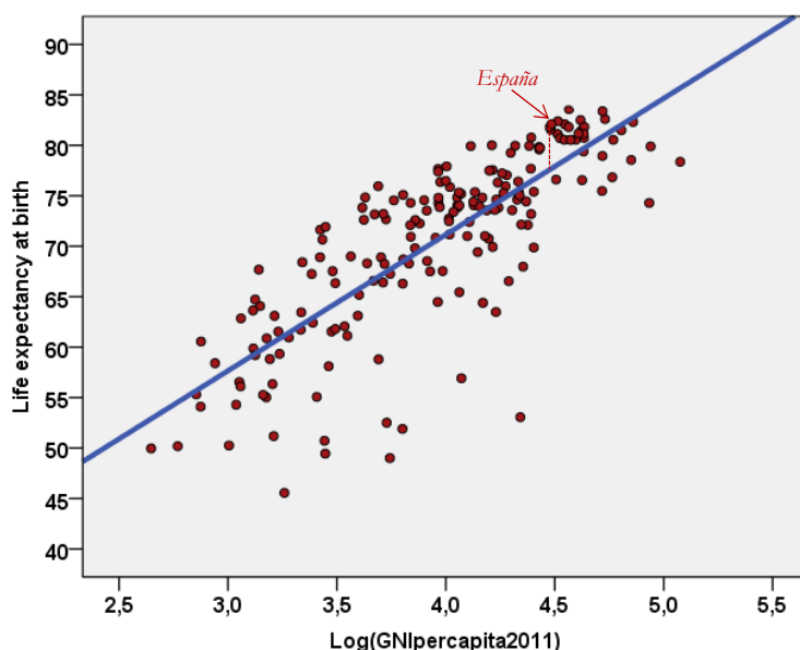
Gráfico III.9.16. Gráfico de dispersión de la regresión entre la Esperanza de vida al nacer y el logaritmo decimal de la Renta per cápita
