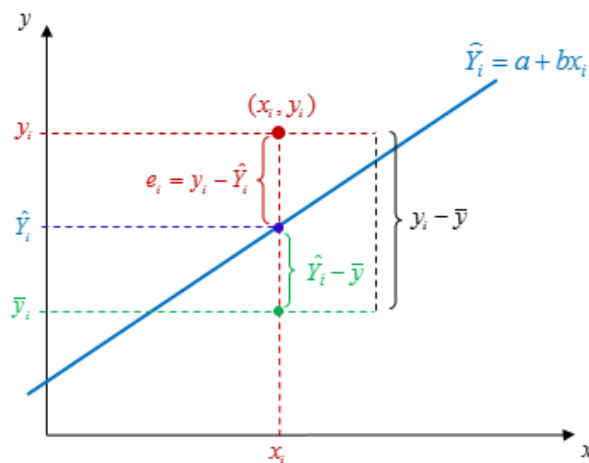
Gráfico III.9.17. Verificación del modelo de regresión
