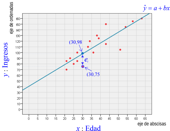
Gráfico III.9.1. Diagrama de dispersión. Nube de puntos y recta de regresión
