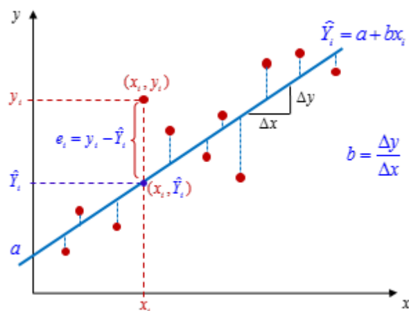
Gráfico III.9.10. Modelo lineal de regresión simple
