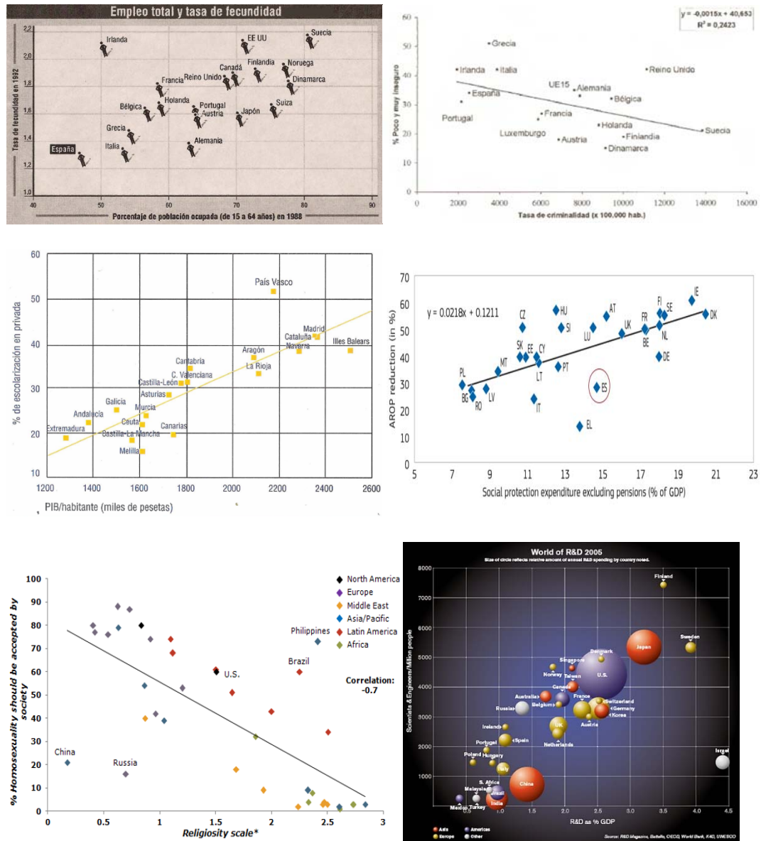
Gráfico III.9.2. Ejemplo de relaciones con gráficos de dispersión
