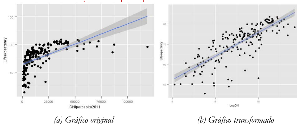
Gráfico III.9.8. Diagramas de dispersión original y transformado entre la Esperanza de vida y la Renta per cápita
