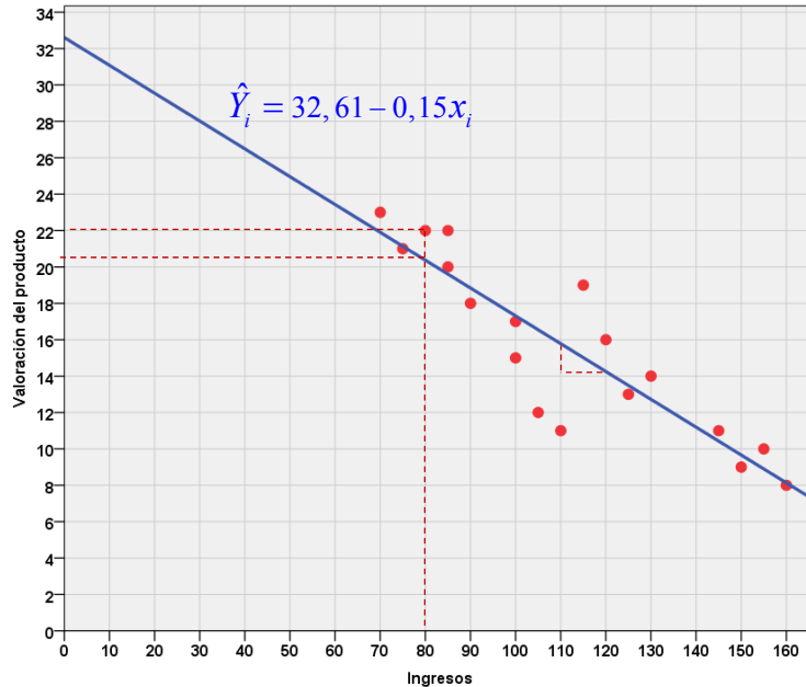
Gráfico III.9.13. Gráfico de dispersión de la regresión entre Valoración e Ingresos
