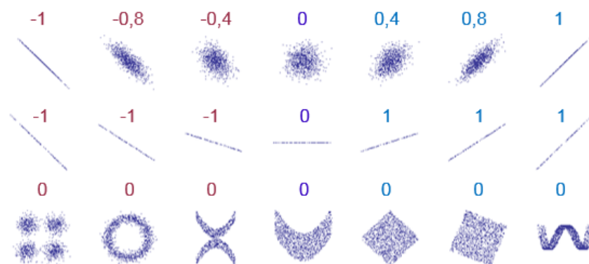
Gráfico III.9.5. Diagramas de dispersión y coeficientes de correlación
