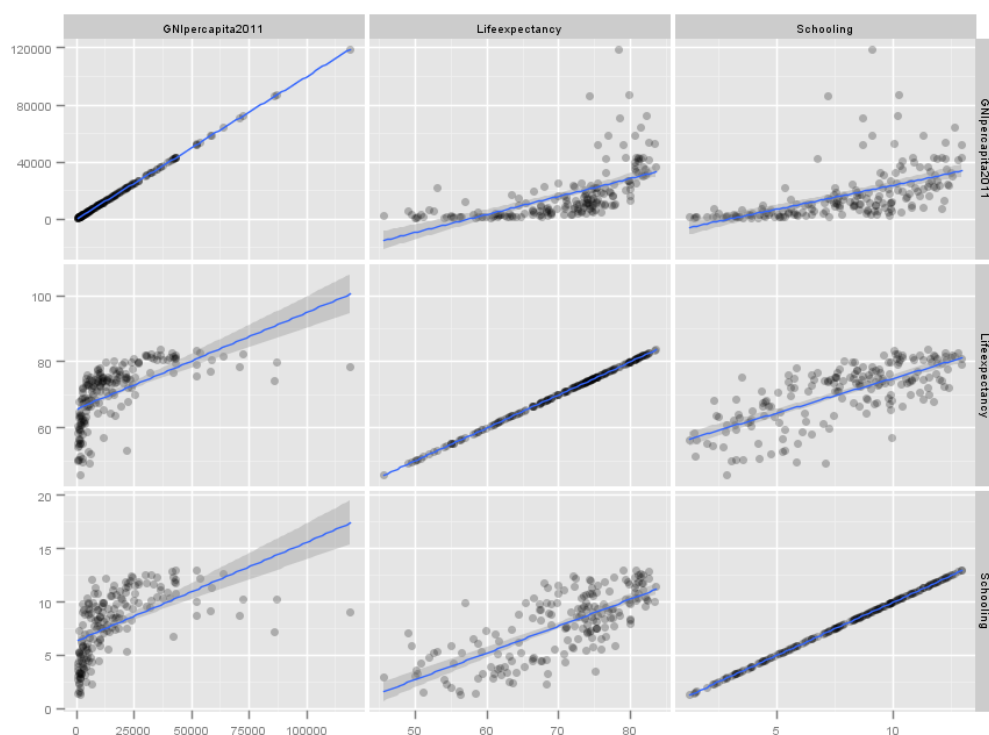
Gráfico III.9.7. Diagrama de dispersión matricial entre la Esperanza de vida, la Renta per cápita y los Años de escolarización de los países del mundo
