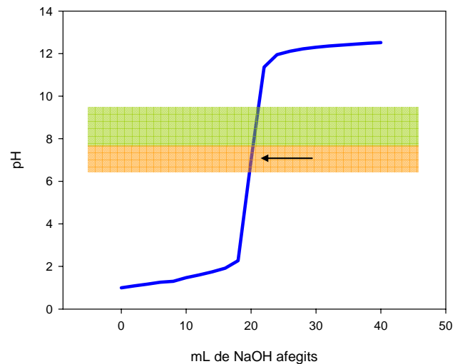
Figura 3. Corba de valoració d'un àcid fort amb una base forta. En verd es representa l'interval de viratge de la fenolftaleïna. Tot i que no conté el punt d'equivalència, l'error que fem és petit degut a que el pendent de la corba és molt pronunciat. El vermell neutre seria en aquest sentit un indicador més adequat. (Podeu consultar ta taula 1).
