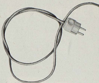
Placa calefactora para madrigueras. Mide 26x34,5 cm. y está construída de fibra de vidrio y fibrocemento; la regulación térmica se produce mediante un termostato electrónico y sonda termostática.
