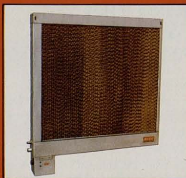
DY-EX PAN. Paneles refrigerantes por evaporación de agua. Varias capacidades, para locales y naves en general. Sistema por depresión.
