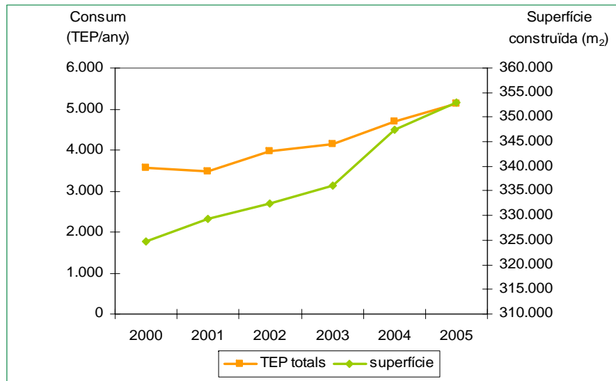
Consum d'energia (gas natural i electricitat) i superfície construïda a la UAB (2000-2005)
