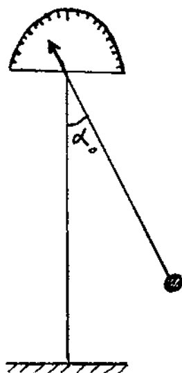
Figura 1 Dispositif expérimental.
