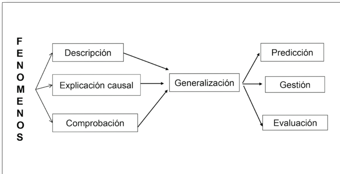
Figura 2. Relación entre los diferentes componentes de la explicación científica (adaptado a partir de Pickett, Kolasa y Jones, 1994).
