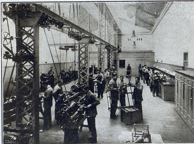
Taller de precisión en el Laboratorio de Aeronáutica, que dirige en Madrid el Sr. Torres Quevedo
