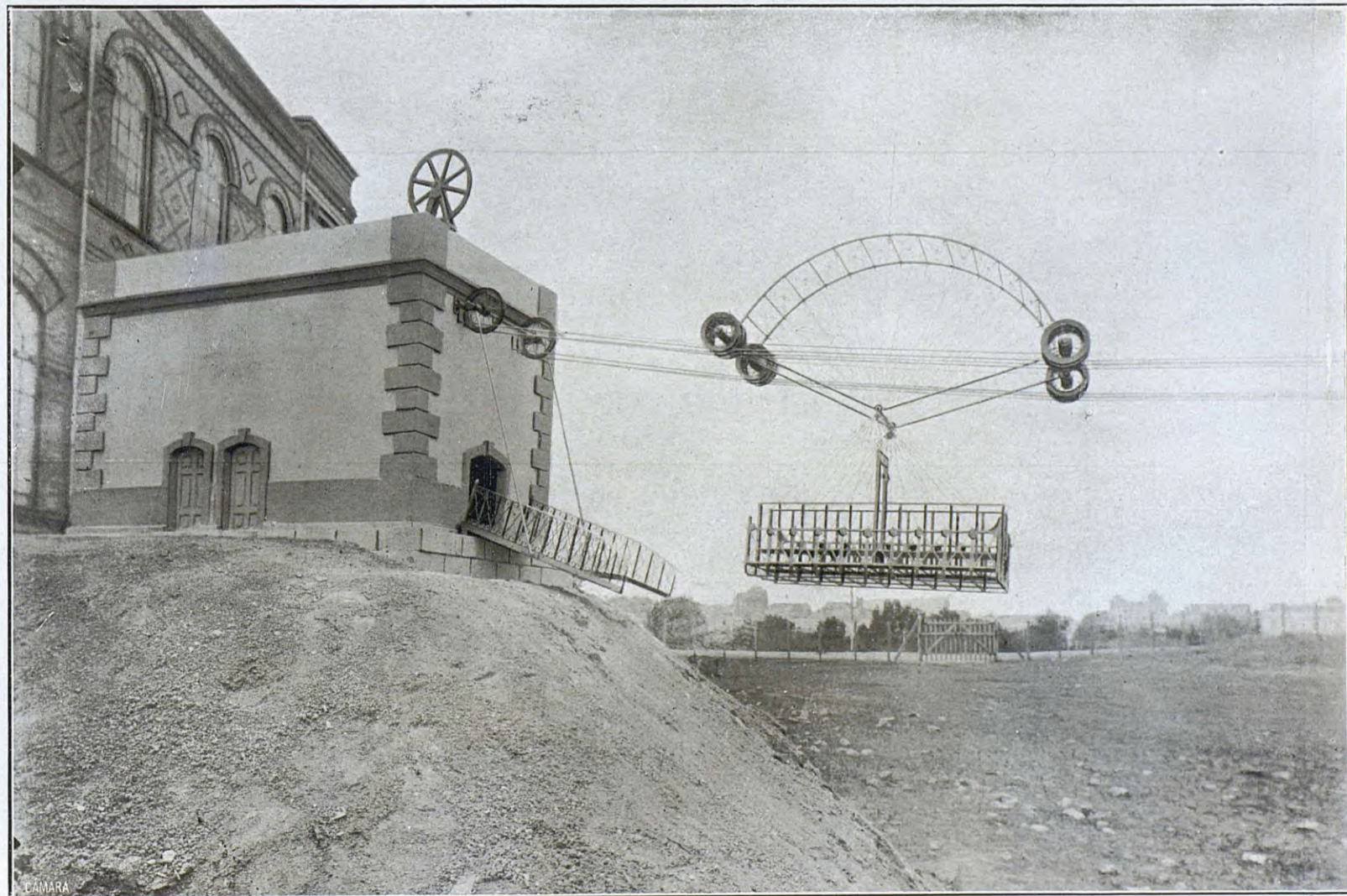
El transbordador funicular Torres Quevedo instalado en el monte Ulía, de San Sebastián
