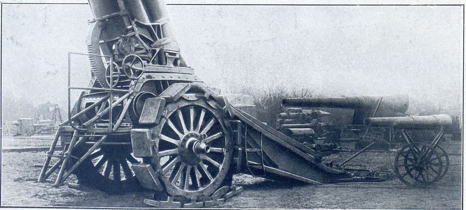
Cañón Howitzer, de sitio, con gran ángulo de fuego. El alcance eficaz es de 7 kilómetros. El proyectil pesa 40 kilogramos y lleva carga de poderosísimos explosivos
