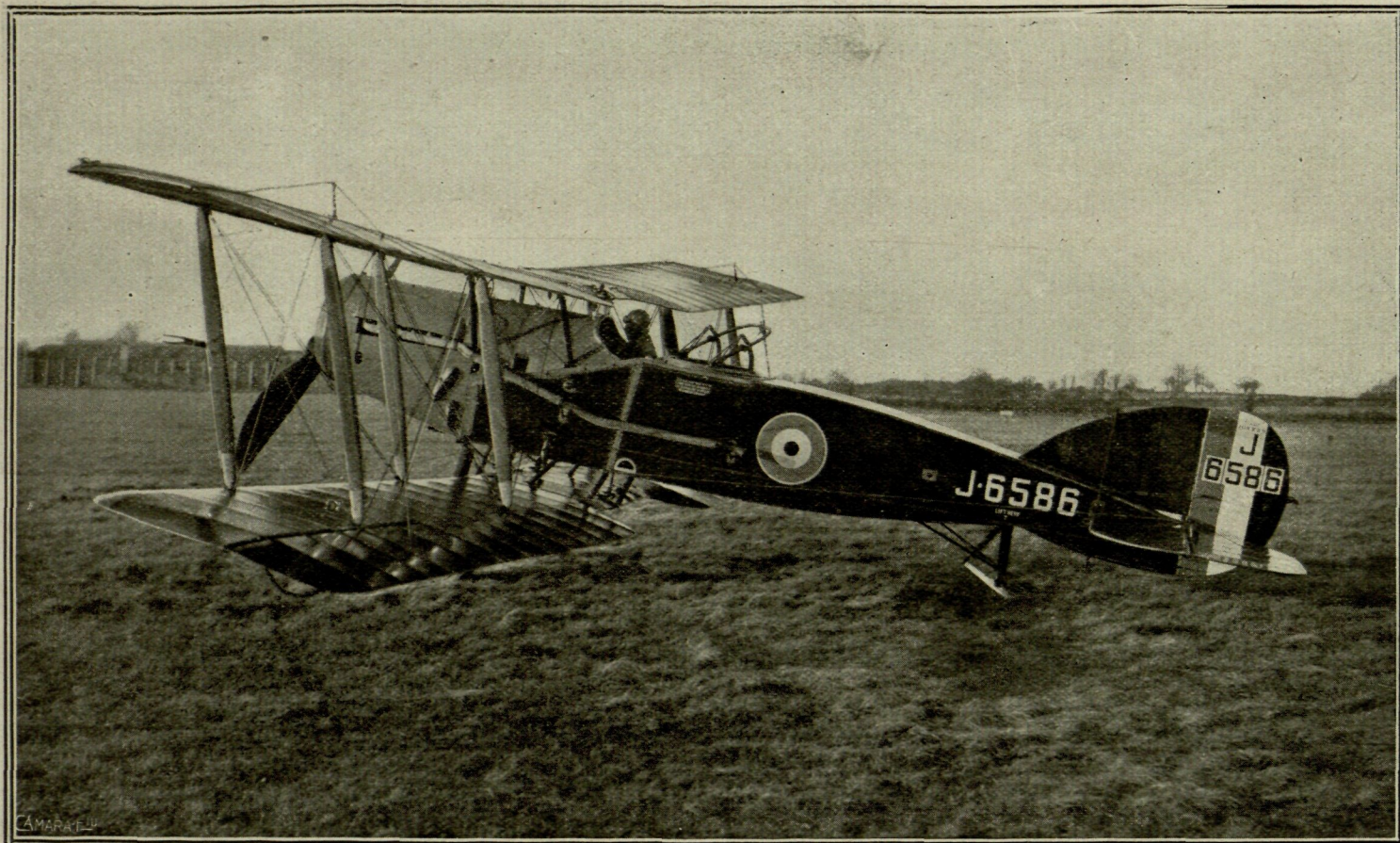
Biplano "Bristol", con motor Hispano-Suiza de 300 HP., modelo de los adquiridos por el Gobierno español para el Ejército á la Compañía Española de Navegación Aérea, S. A., de San Sebastián, representante en nuestro país de la importante Casa inglesa
