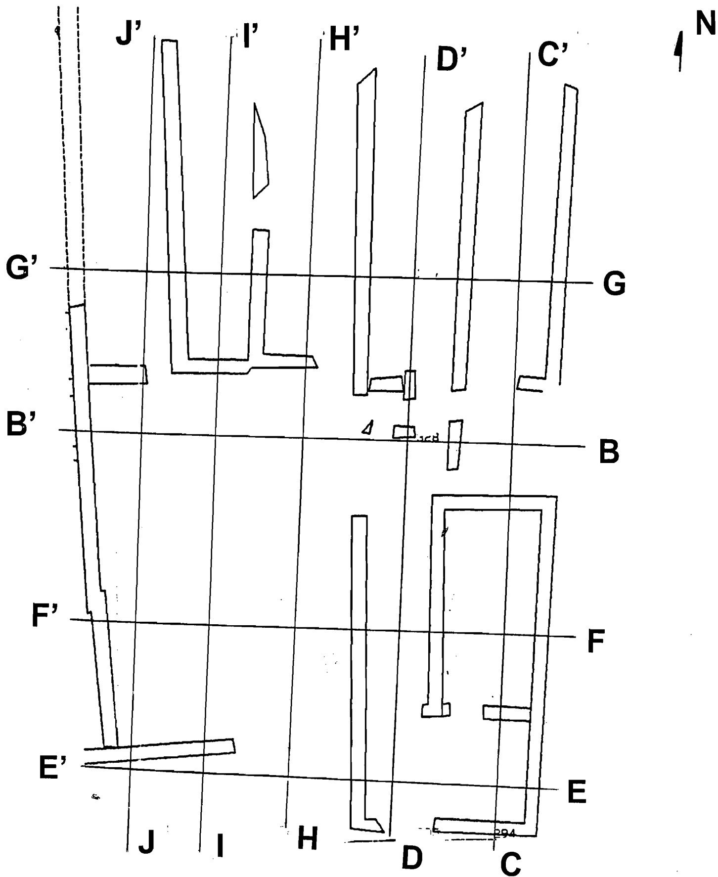
CASTELLET DE BANYOLES TIVISSA (RIBERA D'EBRE) 1999 ZONA 2. EDIFICI 1 SITUACIÓ DE LES SECCIONS 1:100
