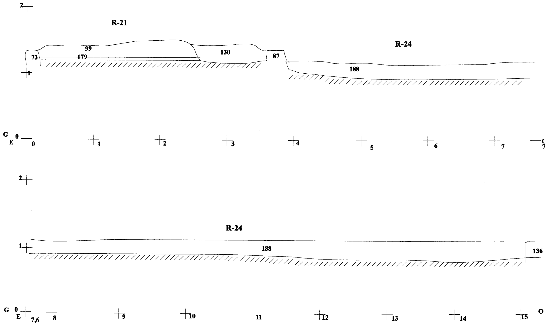
CASTELLET DE BANYOLES, TIVISSA (RIBERA D'EBRE) Campanya 2000 Secció E-O G-G'
