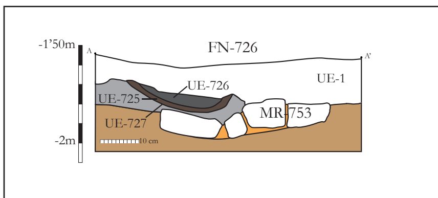
Figura 11. Secció del forn de bronze documentat sobre els nivells ibèrics.
