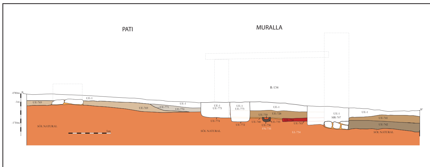
Figura 10. Secció representativa del pati obert i el cos de muralla de compartiments.
